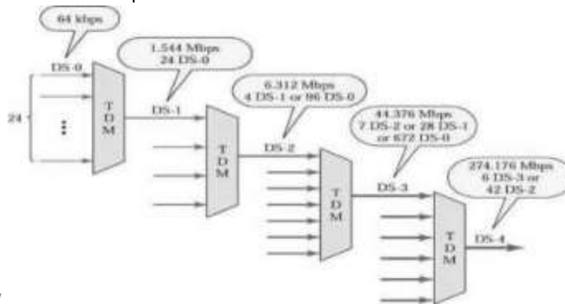
DS-hierarchy
